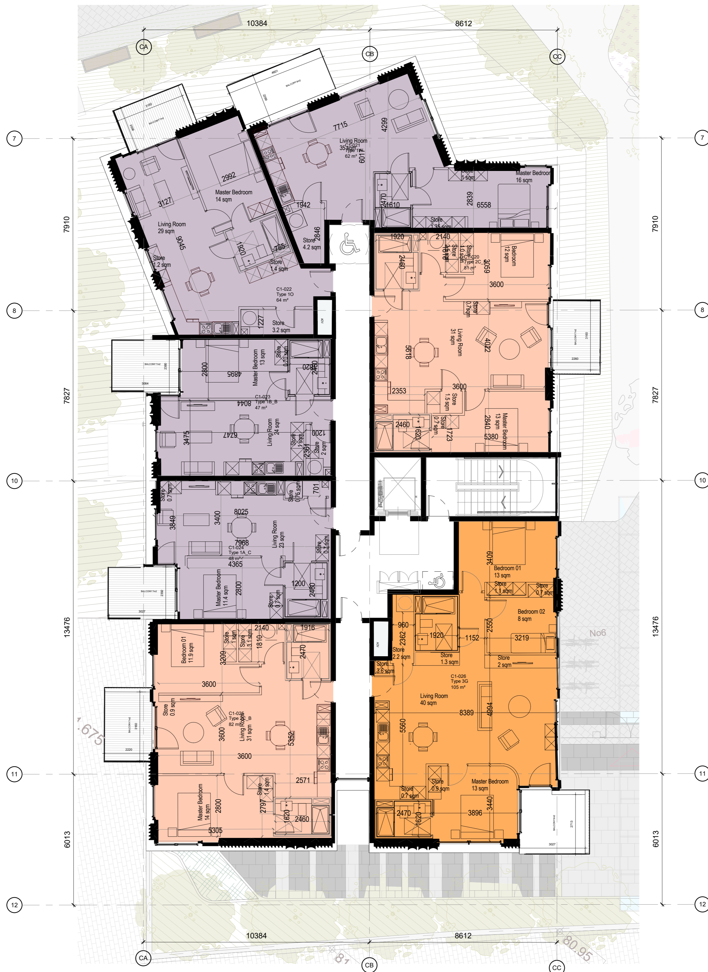
1 03 FFL GA Part V Block C 1 : 100
